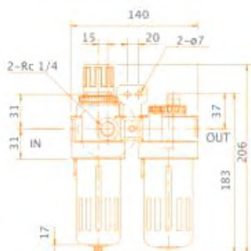
Размеры серии HT-609
