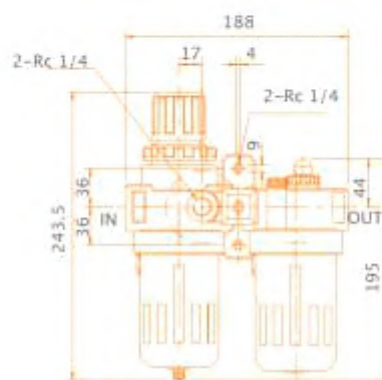
Размеры серии HT-669
